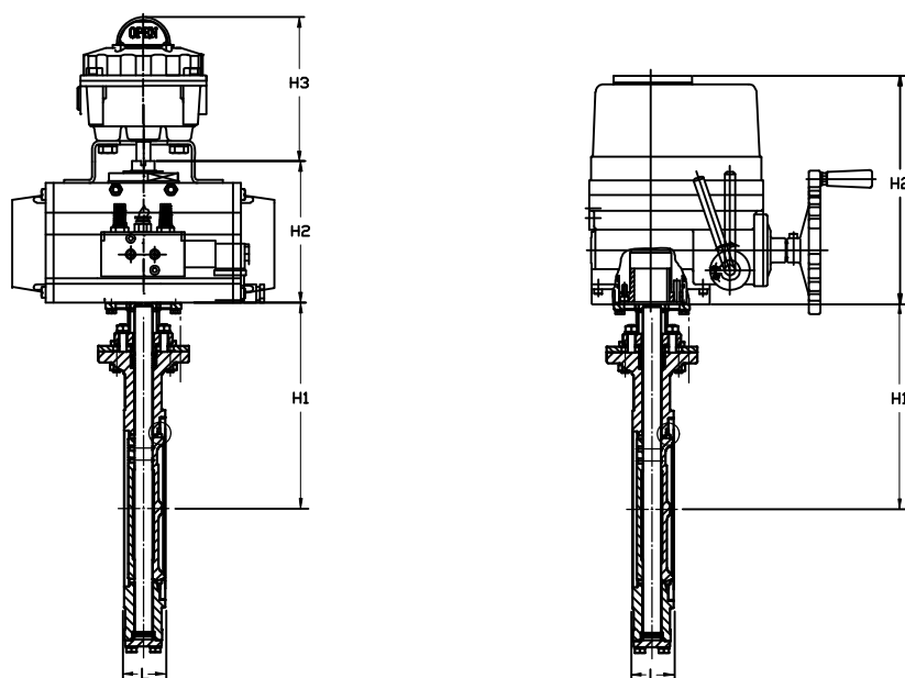
BFV-120A控制蝶閥配置及安裝尺寸表 ( 16KG工作壓力 )
