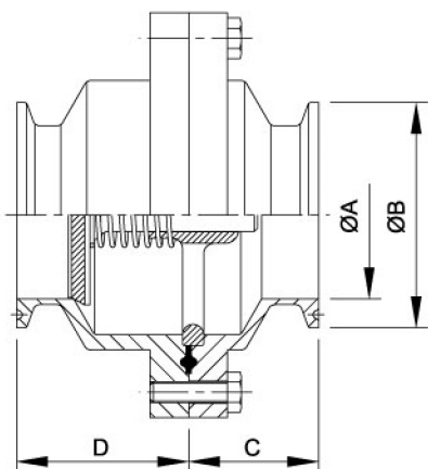
中間法蘭/兩端夾式止回閥
