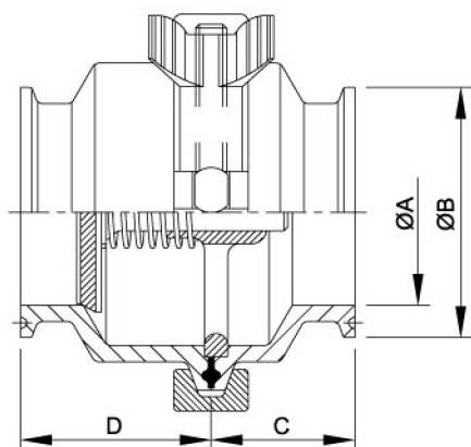
中間夾式/兩端夾式止回閥
