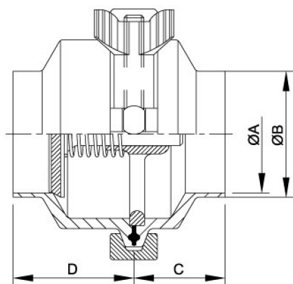
中間夾式/兩端焊接式止回閥
