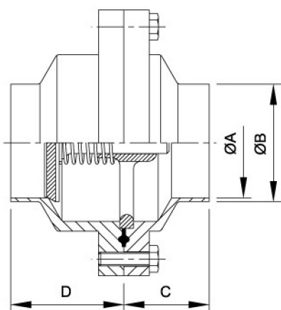
中間法蘭/兩端焊接式止回閥
