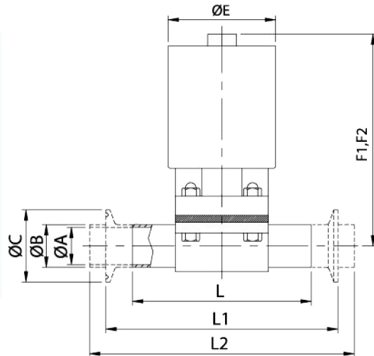
兩通潔淨隔膜閥（手動/氣動）安裝尺寸表
